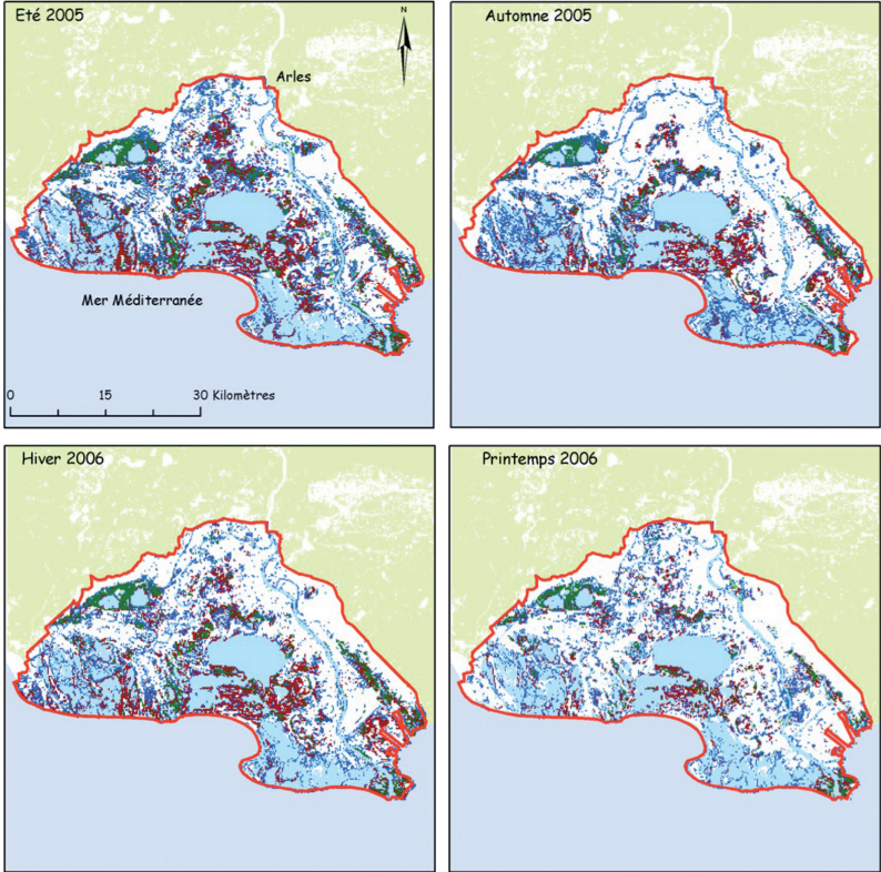
Figure 27. Carte des milieux favorables au développement des gîtes larvaires d' Aedes caspius , en fonction des saisons pour l'année 2005-2006 en Camargue.
