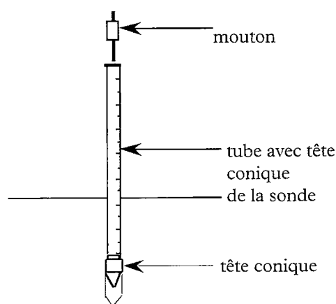
→ Figure 1. Schéma de principe d'une sonde de battage.
