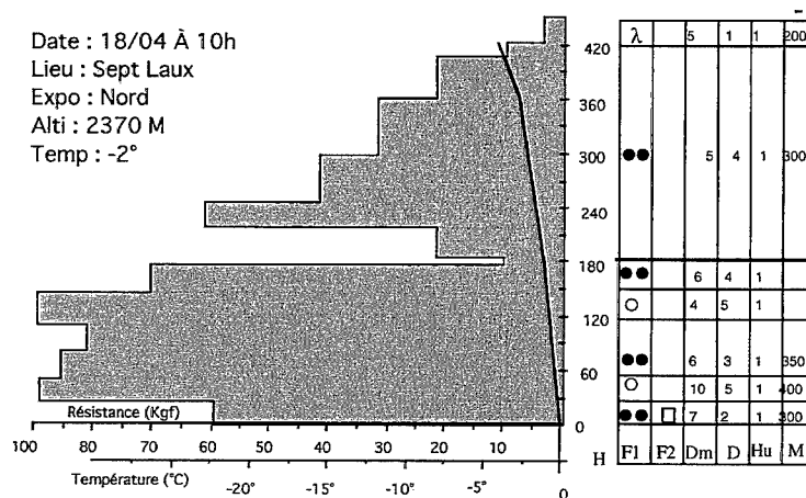
→ Figure 10. Histogramme de résistance au battage et profil stratigraphique d'après un sondage du CEN réalisé le lendemain à l'endroit du décrochement.
