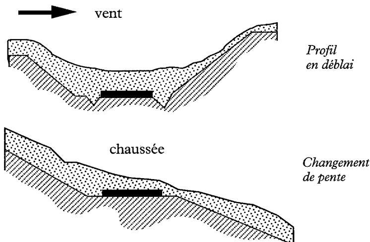
→ Figure 7. Profils propices au développement des congères. D'après [8].
