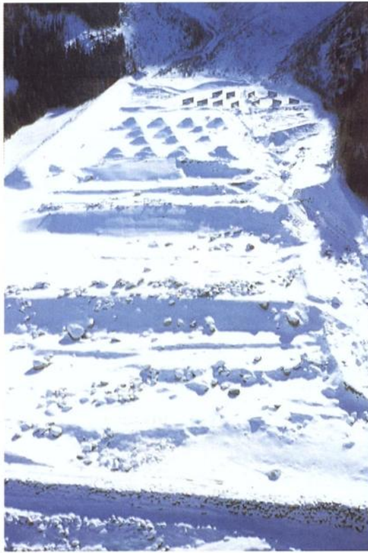
Vue aérienne du dispositif de Taconnaz en février 1992. Le coût a été de l'ordre de 25 millions de francs. Cliché C. Charlier.
