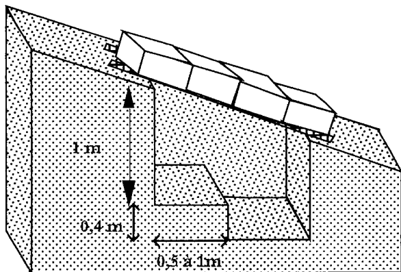
→ Figure 9. Schéma de réalisation du trou dans la neige (banquette et fosse à froid).
