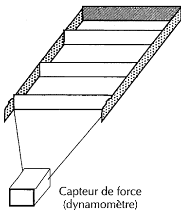
Figure 4 : le cadre de cisaillement est composé d'un cadre rigide maintenant des peignes. On tire, tout en mesurant la force nécessaire à l'aide d'un dynamomètre, sur le cadre placé le long de la couche dont on souhaite étudier les propriétés. On peut mesurer la force de rupture pour différentes charges normales; pour cela il suffit de placer différentes charges de neige dans les espaces entre les peignes. La surface de cisaillement est généralement comprise entre 100 et 500 cm 2 .
