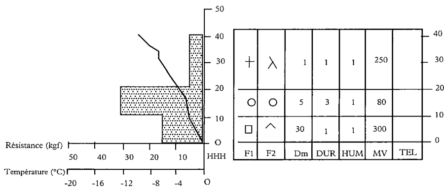
→ Figure 2. Type de représentation préconisé par Météo-France. HHH désigne la hauteur de neige en cm, F1/F2 le type de grains majoritaires/minoritaires, Dm le diamètre moyen, DUR et HUM les indices de dureté et d'humidité, MV et TEL les mesures de masse volumique et de TEL.
