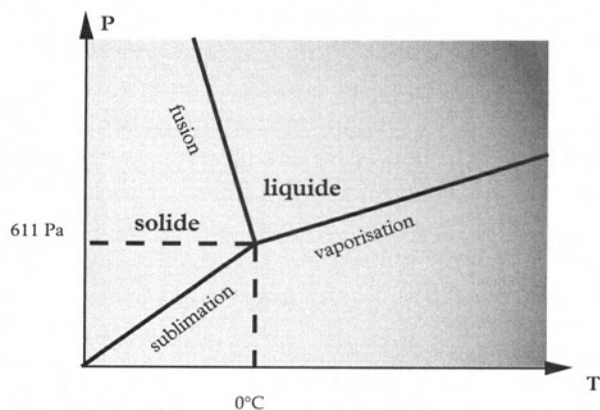
→ Figure 1 : diagramme des phases en fonction de la température (T) et de la pression P. Les coordonnées du point triple sont indiquées.
