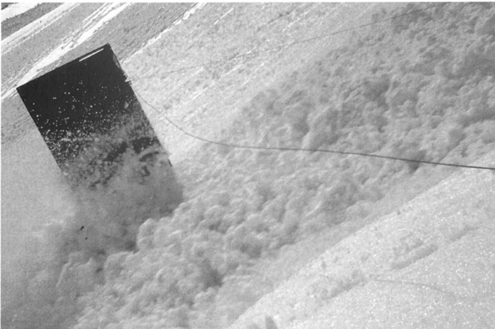
Écoulement dense sur le site expérimental du col du Lautaret (Hautes Alpes). Cliché O. Marco.
