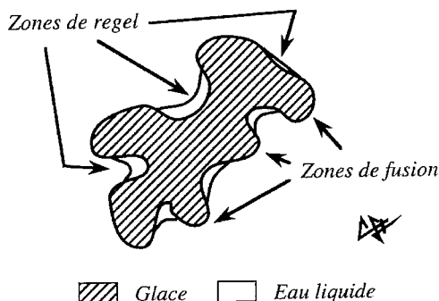
Figure 7. Schéma montrant, pour un grain de neige, les zones de fusion (convexités) et les zones de regel (concavités).
