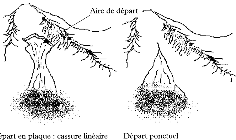
→ Figure 3. Modes de départ : départ en plaque ou ponctuel. L'aire de départ dans le cas d'avalanches avec départ en plaque est assez facile à délimiter.
