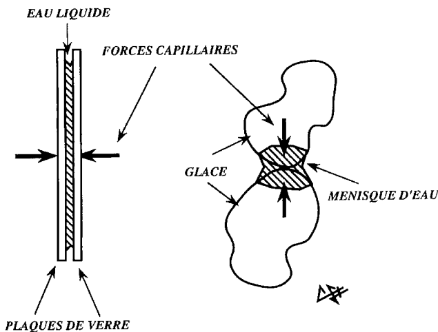
Figure 6. Lorsque l'on accole deux plaques de verre mouillées, on constate qu'il est très difficile de les séparer ensuite. Les forces capillaires se développent au sein du film d'eau liquide et s'exercent sur les plaques. C'est le même phénomène qui se produit lorsque deux grains de neige humides sont en contact. L'eau liquide forme un ménisque autour du point de contact et les forces capillaires tendent à les maintenir accolés.
