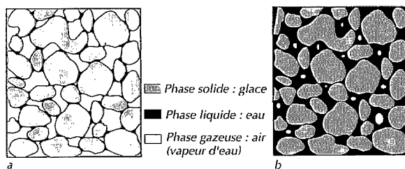
Figure 8. Schéma de la répartition des trois phases de l'eau, dans le cas des faibles TEL (a) et dans le cas des fortes TEL (b).
