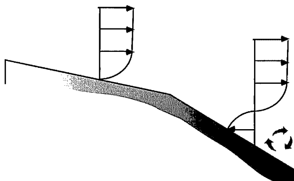
→ Figure 15 : Effet d'un changement de déclivité.
