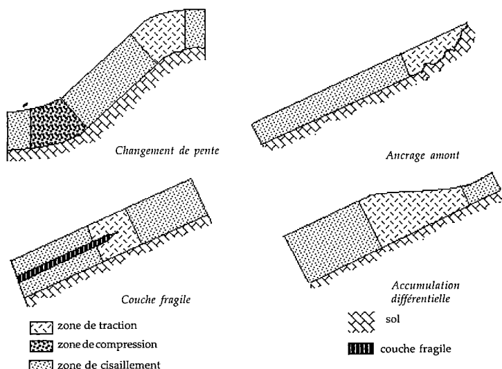
→ Figure 9. Schémas de principe de l'apparition des zones où le cisaillement devient important et conditionne l'instabilité éventuelle du manteau.
