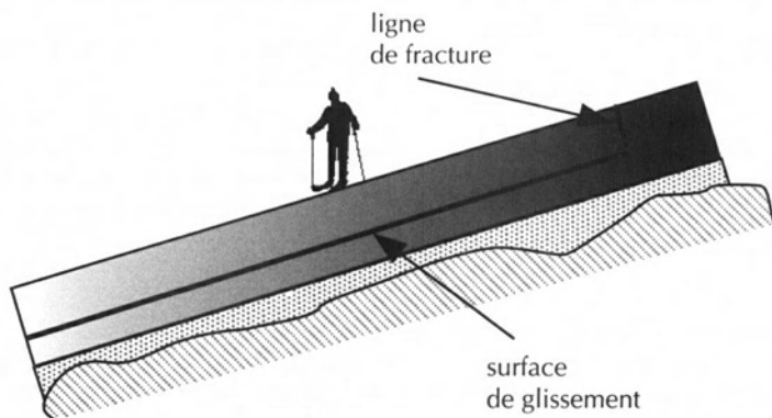
→ Figure 15. La plaque est mise en mouvement après la rupture par traction le long de la ligne de fracture et par cisaillement sur la surface de glissement. La rupture initiale (primaire) peut être selon les mécanismes l'un ou l'autre de ces processus.
