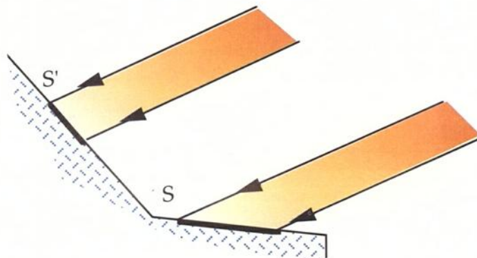
→ Figure 5. Le flux est la quantité de chaleur reçue par unité de surface ; il dépend de l'orientation de la surface par rapport à la direction du rayonnement solaire : le flux est maximal lorsque la surface est perpendiculaire à cette direction.
