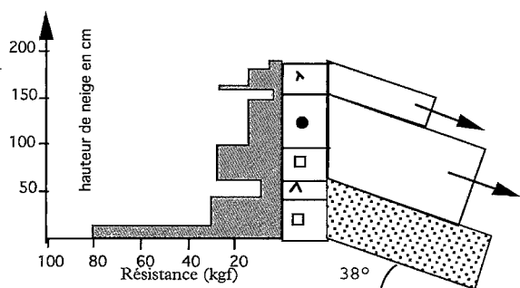
→ Figure 12. Profil simplifié du manteau neigeux lors de l'accident du Piz Ucello, région de San Bernadino (Suisse) le 5 février 1990 (voir récit § 3.3.2). Le coin suisse donne un indice de risque d et la surface de glissement est l'interface entre la couche de neige fraîche et la première couche de grains fins. La surface de glissement de l'avalanche est une dizaine de centimètres au-dessous (interface gobelets/grains fins) [52].
