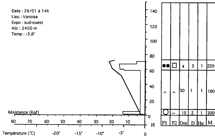
→ Figure 4. Profil réalisé dans le massif de la Vanoise par beau temps le 26 janvier à 14 h à 2450 m. Le profil met en évidence l'existence d'une plaque de faible épaisseur (10 cm), composée de grains fins (neige légèrement ventée?) et de grains à faces planes (métamorphose de gradient moyen due aux conditions anti-cycloniques régnant depuis plusieurs jours).
