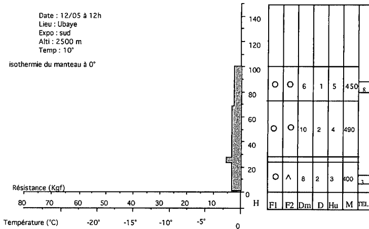
→ Figure 5. Profil réalisé dans la vallée de l'Ubaye par beau temps le 12 mai à 12 h à 2500 m d'altitude. L'ensemble du manteau est de faible cohésion et largement humidifié. La TEL est supérieure à 6 % sur la quasi totalité du manteau, ce qui indique le "pourrissement" de l'ensemble du manteau, qui est déjà ancien (la masse volumique approche dans la partie médiane les 500 kg/m 3 ). Le risque d'avalanche (mobilisant de la neige lourde) n'est pas négligeable. D'après [3].
