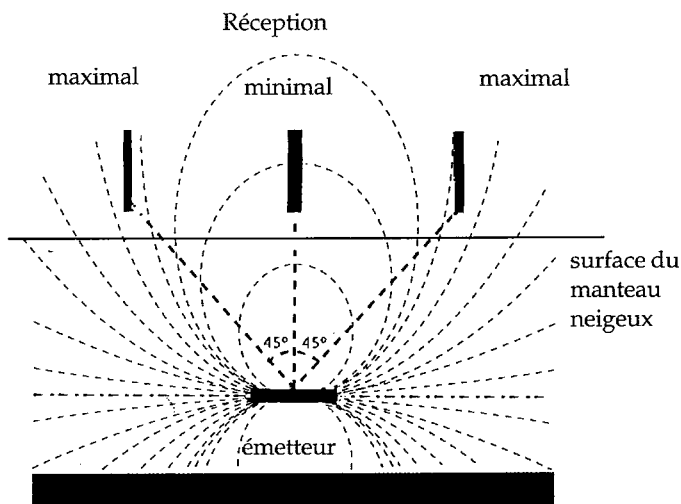
→ Figure 16. Cas où l'ARVA se situe au milieu des deux extrema. Un cas analogue se produit lorsque l'appareil est placé verticalement.
