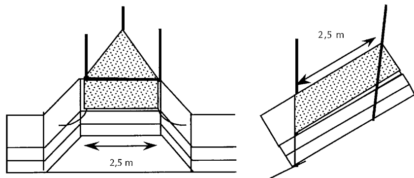
→ Figure 6. Dimensions d'un coin suisse. D'après [45].
