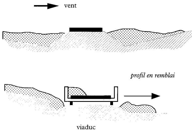
→ Figure 8. Aménagements en vue de réduire les congères. D'après [8].
