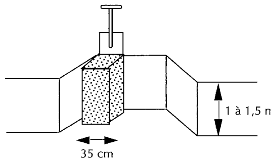
→ Figure 15. Dimensions du test de la pelle selon les normes américaines (voir aussi méthode de Faarlund, chapitre 4, § 2.2.1.).
