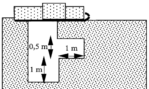
→ Figures 10 et 11. Deux types d'abri : banquette et igloo creusés dans la neige. C'est la tranchée qui sert de fosse à froid.
