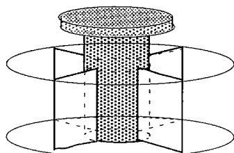
Figure 3 : scissomètre.
