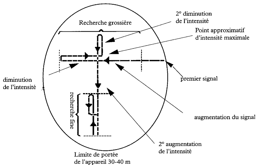
→ Figure 15. Recherche par angles droits.
