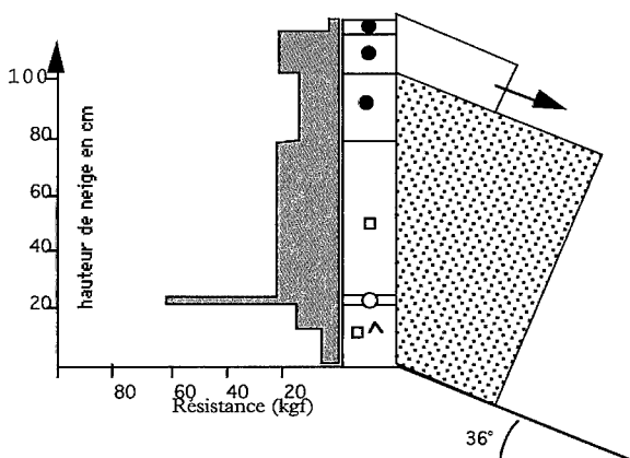
→ Figure 13. Profil simplifié et essai de coin suisse (degré d) le 28.11.92 au Radüner Rothorn (Suisse) à 2880 m d'altitude [52].
