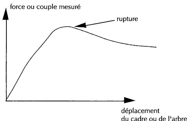
Figure 5 : la détermination de la résistance au cisaillement se fait en mesurant la force (ou le couple) à la rupture. Généralement, la rupture se traduit dans un diagramme force-déplacement (ou couple-rotation) du cadre par l'existence d'un maximum. Le passage de la valeur de la force maximale à la valeur de la résistance fait généralement appel à des facteurs de correction, qui varient selon les auteurs.
