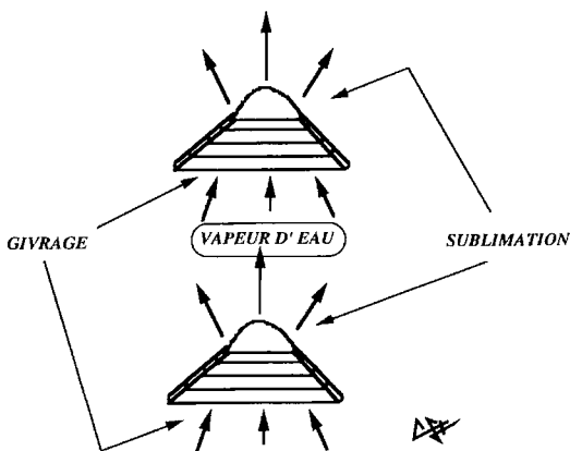
Figure 5. Schéma de formation des gobelets.
