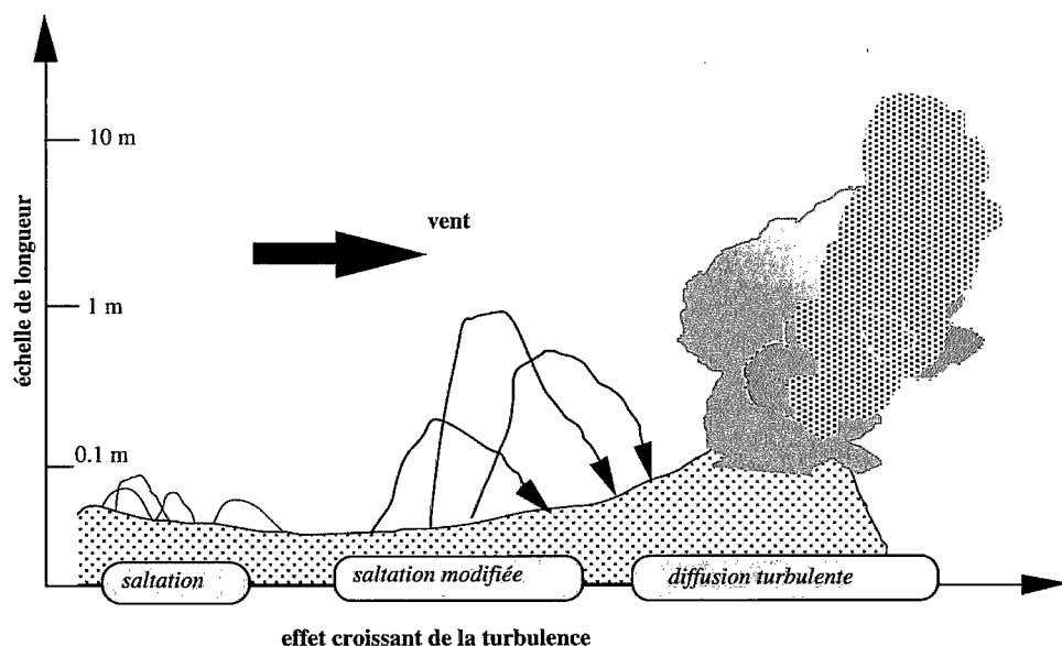
→ Figure 13. Les principaux modes de transport de neige par le vent et leur échelle de longueur (hauteur de l'écoulement de neige reprise).
