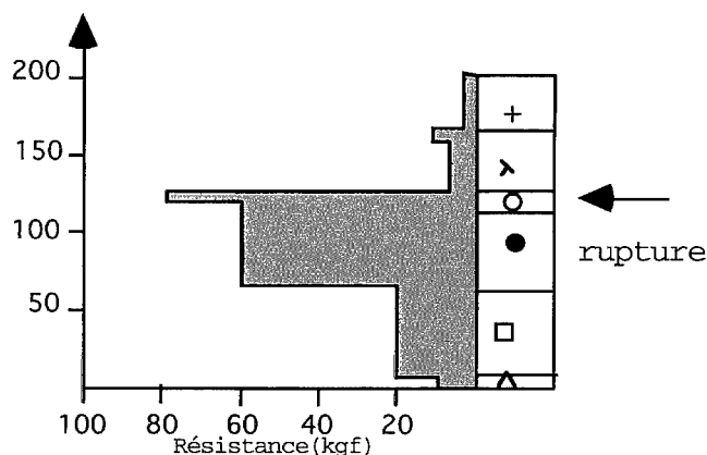
→ Figure 9. Profil simplifié de Rosswald. Le décrochement a affecté la neige fraîche dans son intégralité (épaisseur supérieure 70 cm), le glissement se faisant sur la croûte de regel [1].
