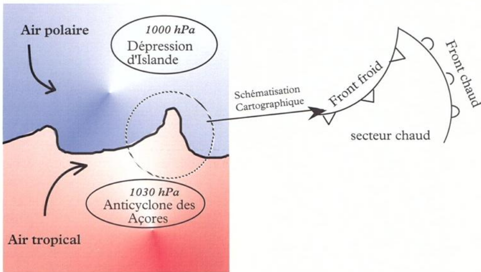
→ Figure 6 : la perturbation née de la zone de contact (rencontre des masses d'air tropical et polaire) provoque un enroulement en spirale caractéristique sur les vues de satellite. D'après [1].
