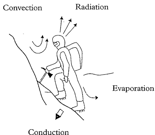
Figure 1 : transferts de chaleur.
