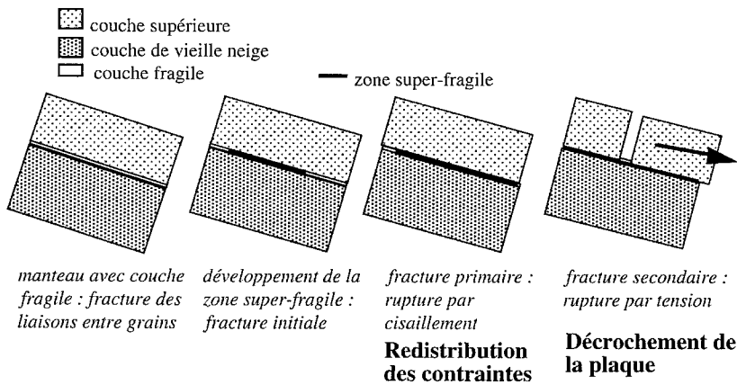
→ Figure 19. Les différentes étapes d'une rupture amenant à un départ en plaque : la rupture de la surface de frottement au niveau de la couche fragile provoque une redistribution soudaine des contraintes.
