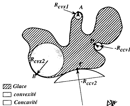
Figure 1. Schéma explicatif des rayons de courbure :
