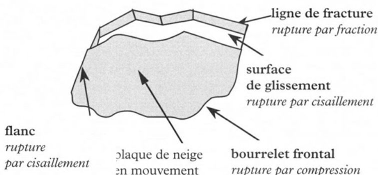
→ Figure 14. Terminologie des ruptures. Les frontières de la plaque de neige sont définies par la rupture de la couche déclenchée, qui se fait en une succession d'étapes dont l'ordre dépend du mécanisme.
