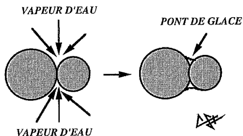
Figure 3. Schéma explicatif du phénomène de frittage. La concavité autour du point de contact entre les deux grains est le siège de la condensation solide de la vapeur d'eau.
