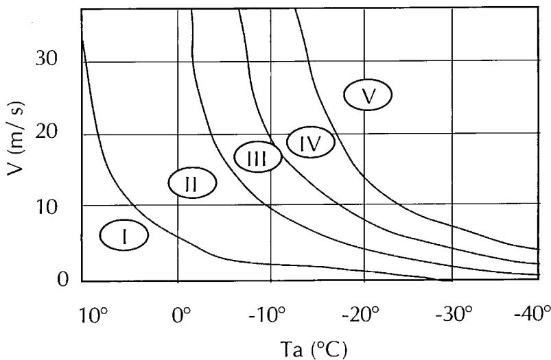
Figure 2 : index Windchill. D'après [5]. Sensation de froid en fonction de la température de l'air ( T_a ) et de la vitesse du vent ( V ).
