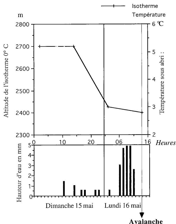
→ Figure 21. Résumé des conditions météorologiques précédant l'avalanche du tunnel du Mont-Blanc (cf. § 1.1.3.) : isotherme 0 °C (d'après radiosondages de Lyon et Payerne), température (station Nivose des Aiguilles-Rouges, 2 330 m), précipitations (recueillies à Chamonix). L'avalanche a eu lieu le 16 mai 1983 à 14 h 10.
