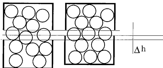
→ Figure 20. Le cisaillement d'un échantillon granulaire lâche provoque une réorganisation des particules et donc une légère diminution de volume (mais pas un affaissement). Dans le cas de gobelets, cette diminution de volume peut être accrue par l'écrasement des cristaux.
