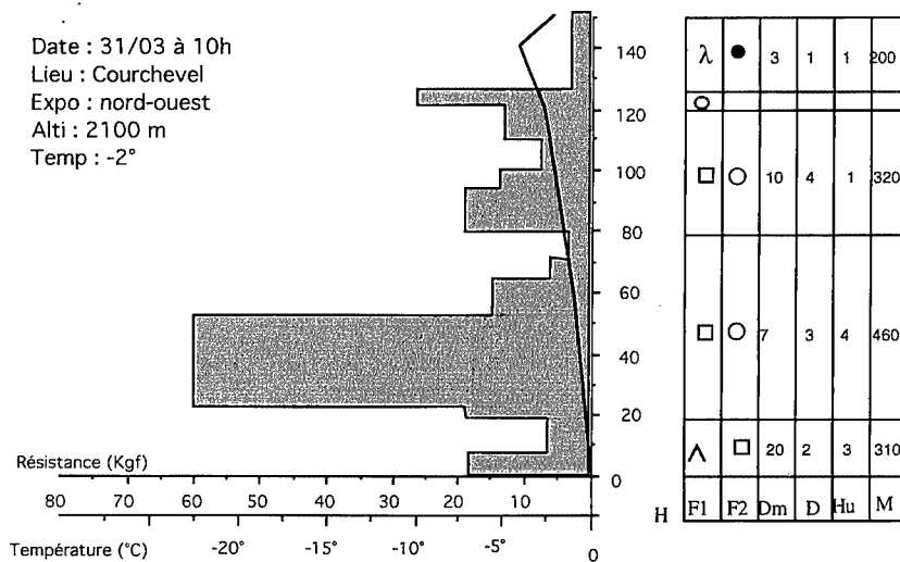
→ Figure 8. Profil simplifié du battage d'après le poste d'observation nivo-météorologique de Biolley-Verdons (Courchevel) du 31 mars 1992. D'après document CEN.
