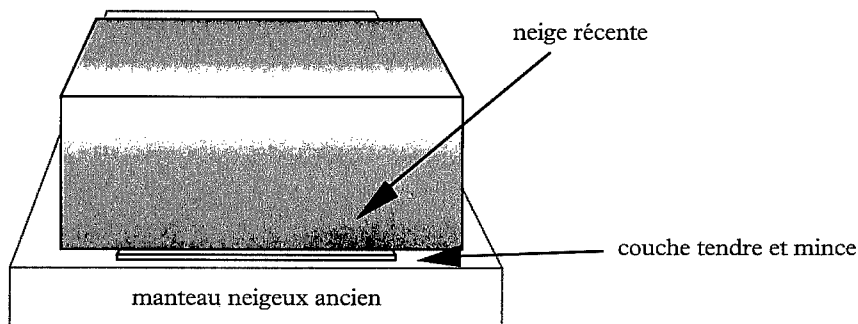
Figure 2. Couche tendre et mince sous la neige récente : le piège !
