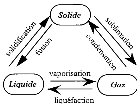
→ Figure 2 : désignation des différents types de changements de phase selon le sens de ce changement.
