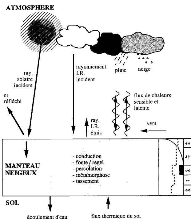
Figure 10. Les termes du bilan énergétique du manteau neigeux.
